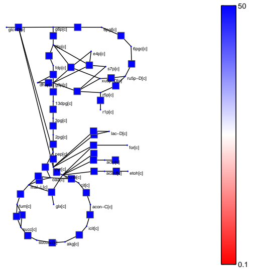
(d) Thermodynamic forces (kJ/mol)
