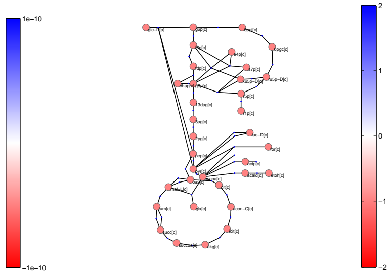
(d) Thermodynamic forces (kJ/mol)
