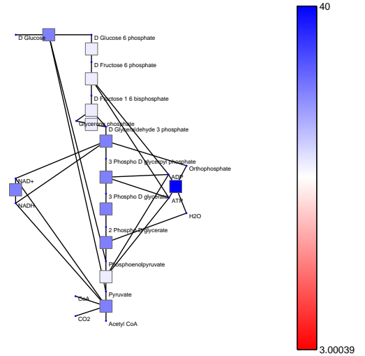
(d) Thermodynamic forces (kJ/mol)
